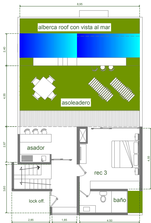
planta alta PH
