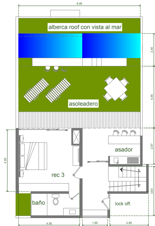
planta alta PH
