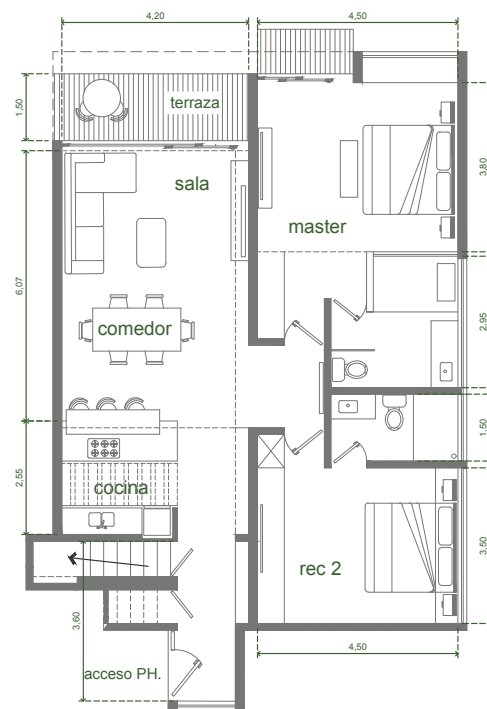
planta baja PH
